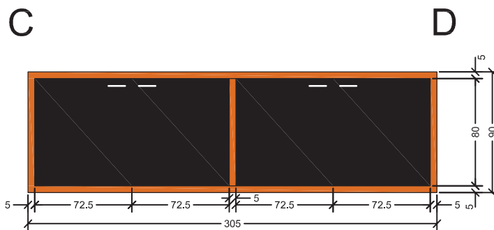
Widok C-D
