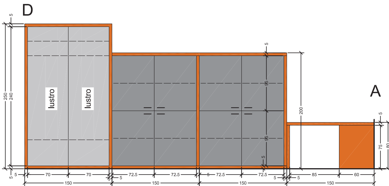
Widok D-A
