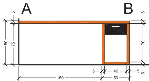
Widok A-B
