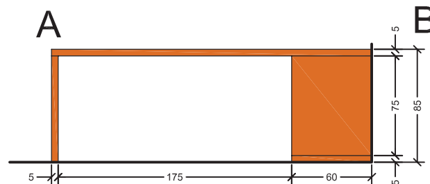
Widok A-B
