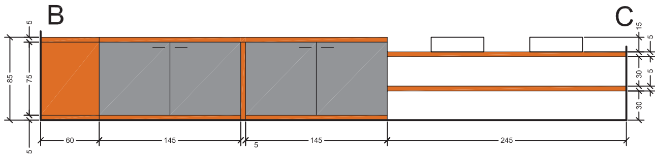
Widok B-C
