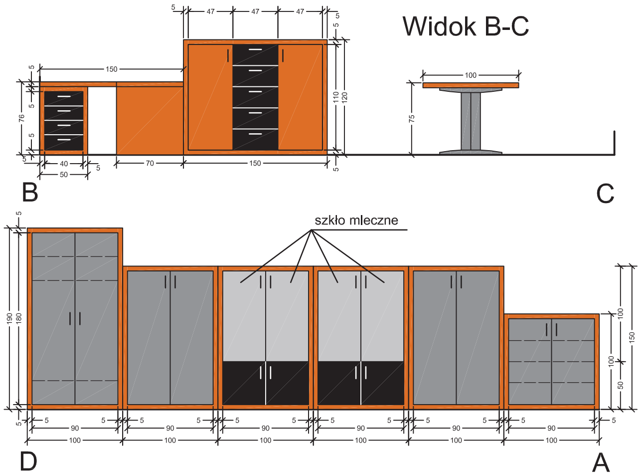
Widok D-A
